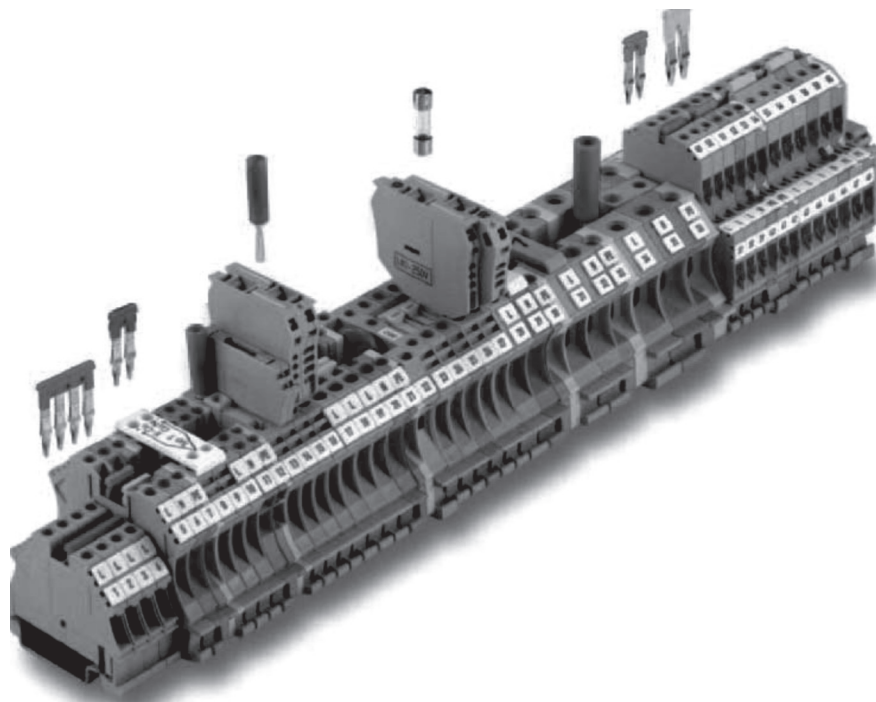
Рисунок 6.14 – Сборка из наборных зажимов
