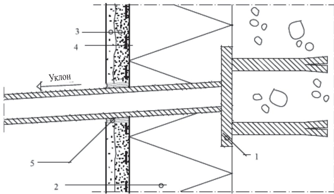
Рисунок 9.8 – Устройство системы в месте устройства воздухопроводов
