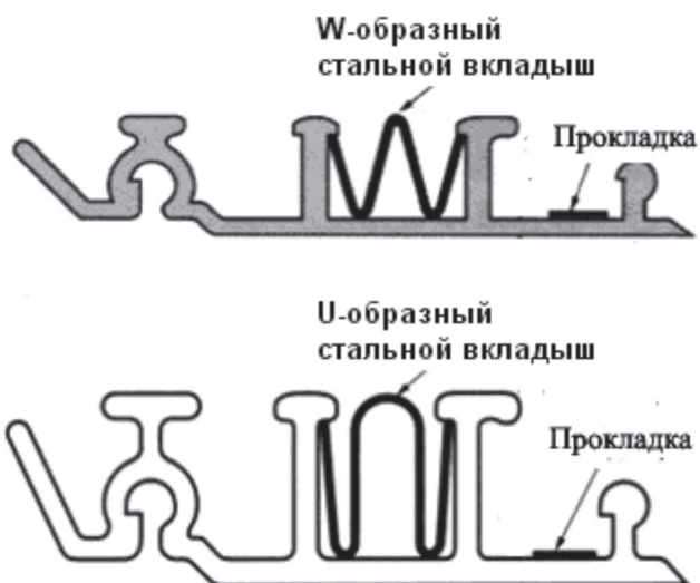
а) Варианты формы сечения ПВХ-профиля
