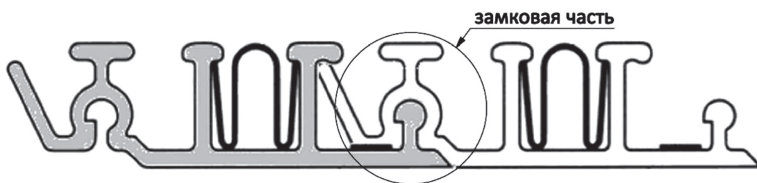
б) Способ скрепления витков профиля между собой
