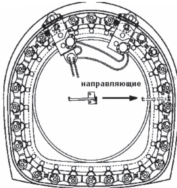
Рисунок 14 – Монтаж направляющей
