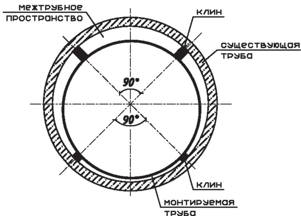
Рисунок 3 – Расположение клиньев
