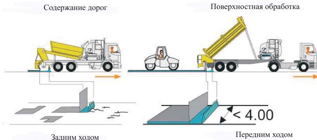
Рисунок 6.2 – Принципы работы машин для поверхностной обработки
