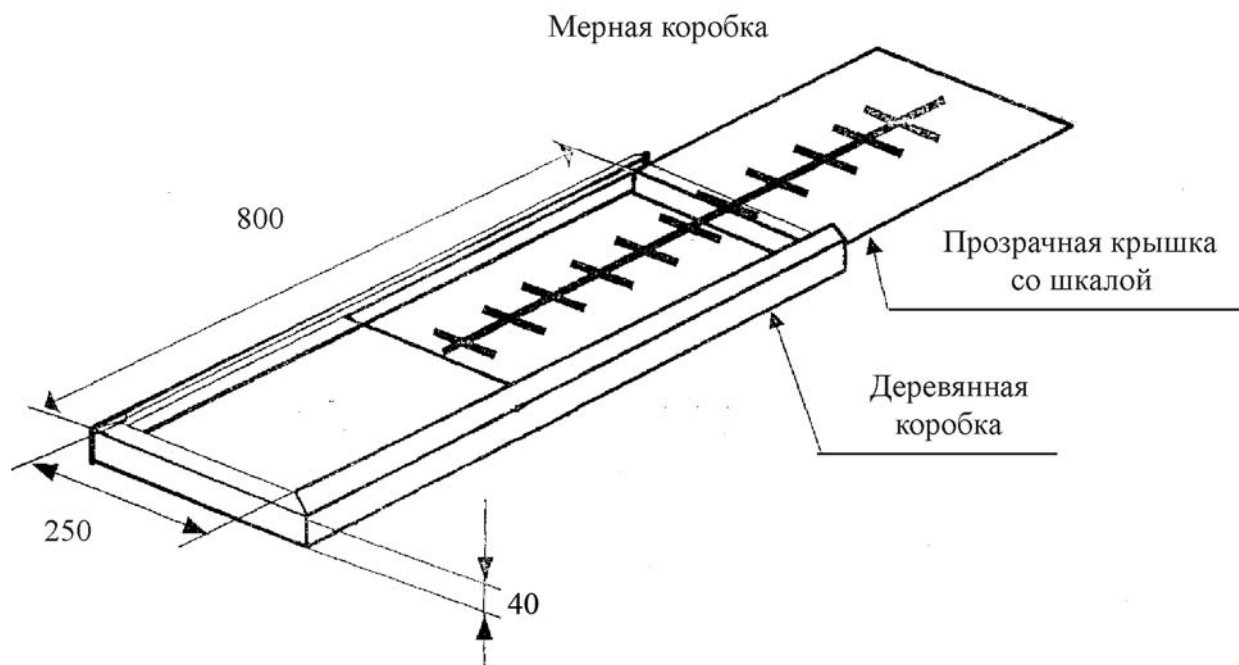
Рисунок М. 1 – Размеры мерной коробки (мм)
