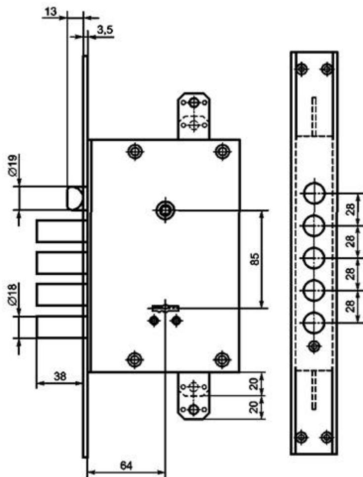
Рисунок Б.6 - Пример сувальдного врезного замка типа ЗВ11
