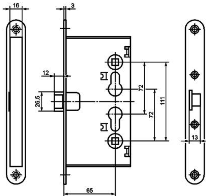
Рисунок Б.12 - Пример замка для противопожарной двери
