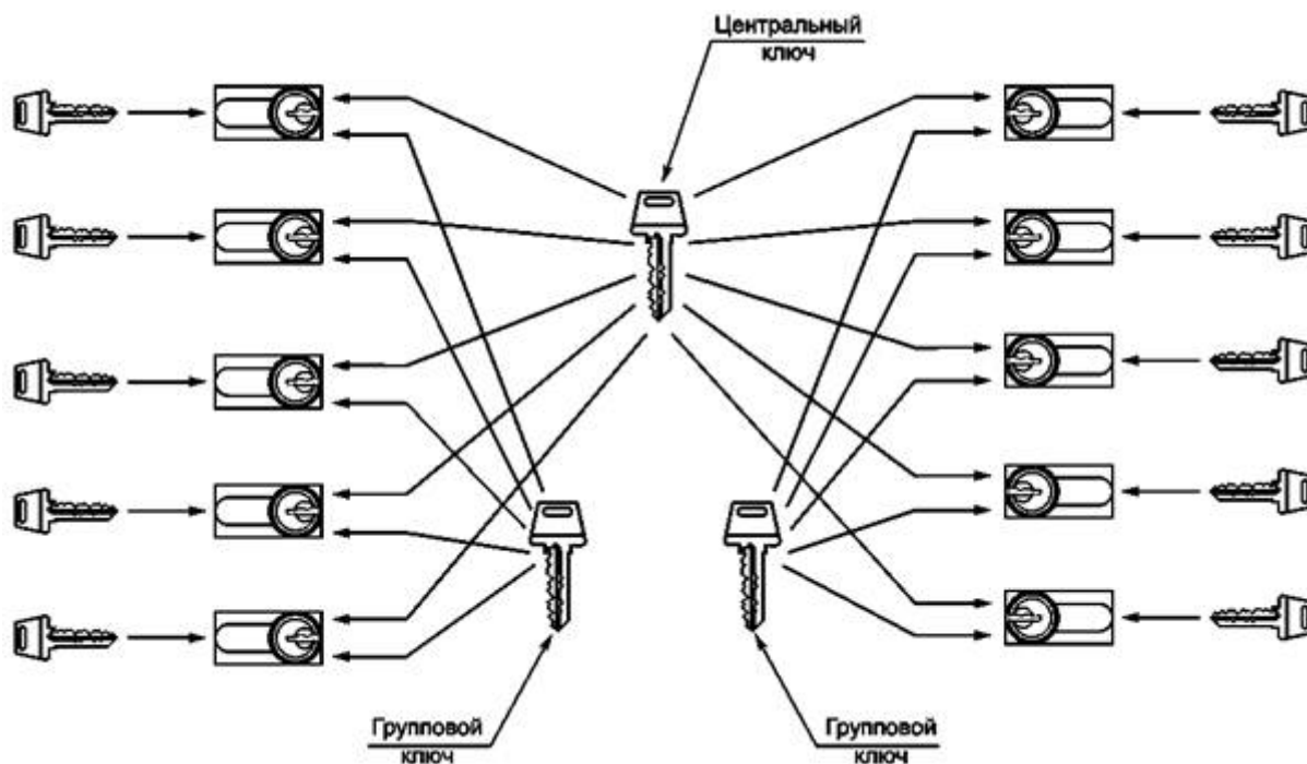
Рисунок А.3 - Система цилиндрических механизмов с групповым ключом - группа механизмов, каждый из которых можно открывать и закрывать как собственным ключом, так и групповым ключом, свойственным для данной группы
