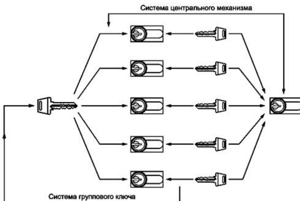
Рисунок А.6 - Смешанная система цилиндрических механизмов - система, представляющая собой соединение систем механизмов цилиндрических с групповым
