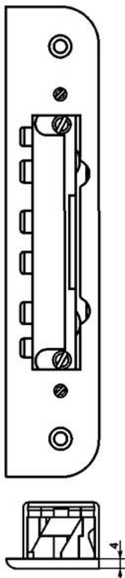
Рисунок Б.17 - Пример усиленной запорной планки коробчатой формы
