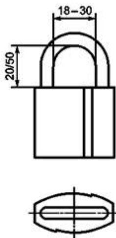
Рисунок Б.13 - Пример навесного замка типа ЗНВ1
